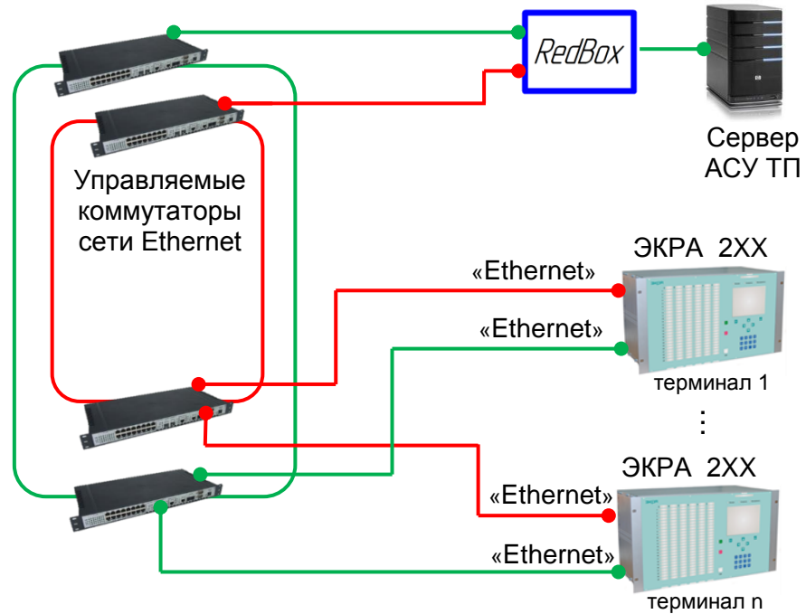
Рисунок 10 – Типовая схема интеграции терминала в резервированную сеть Ethernet по PRP протоколу
