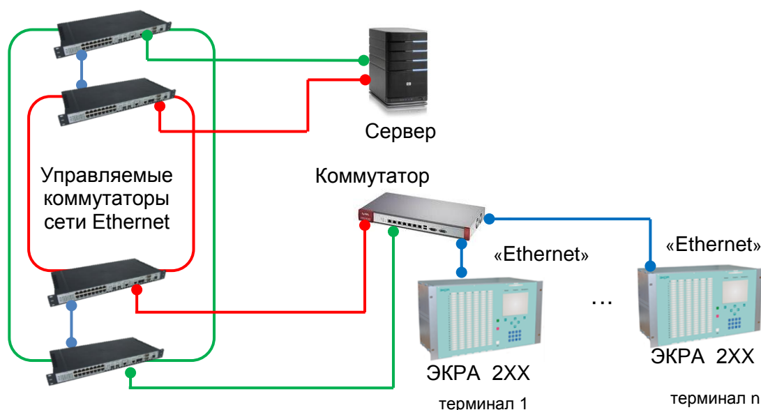
Рисунок 9 – Типовая схема интеграции терминала по RSTP протоколу в резервированную сеть Ethernet на уровне коммутатора
