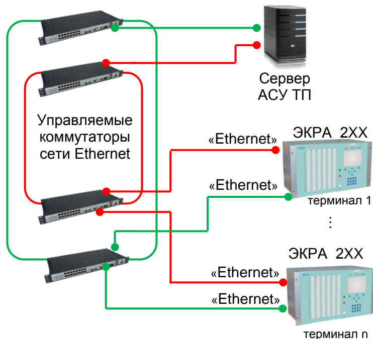
Рисунок 7 – Типовая схема интеграции терминала в резервированную сеть Ethernet по LinkBackup технологии
