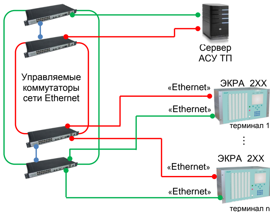
Рисунок 8 – Типовая схема интеграции терминала в резервированную сеть Ethernet по RSTP протоколу
