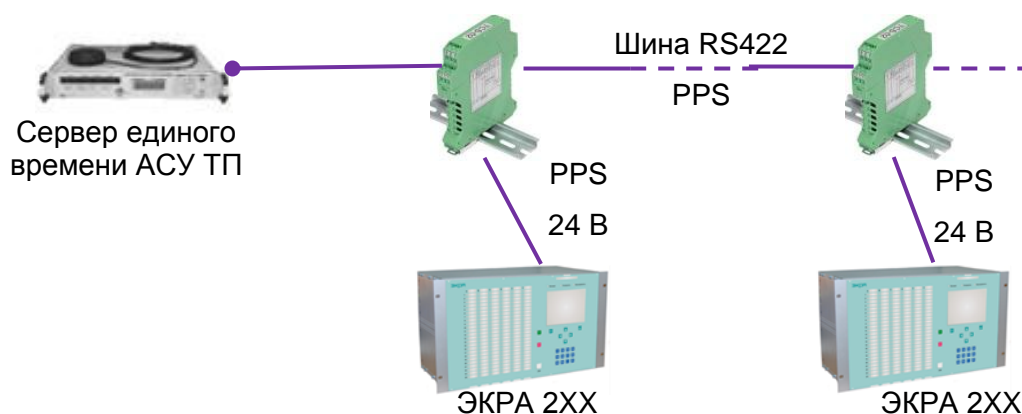
Рисунок 12 – Типовая схема подключения терминала к серверу единого времени АСУ ТП по шине RS422 PPS
