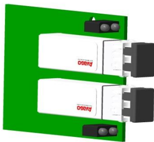
Рисунок Б.4 – Разъем LC интерфейса Ethernet (оптический)
