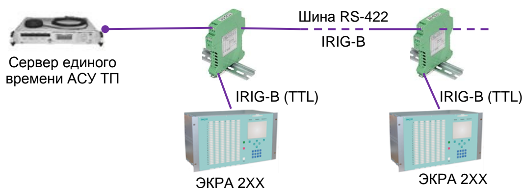
Рисунок 14 – Типовая схема подключения терминала к серверу единого времени Параметры настройки синхронизации времени
